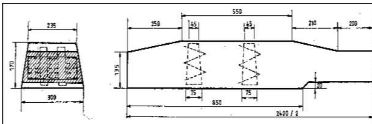
„T” – jelű vasbetonalj (1961-1965)
