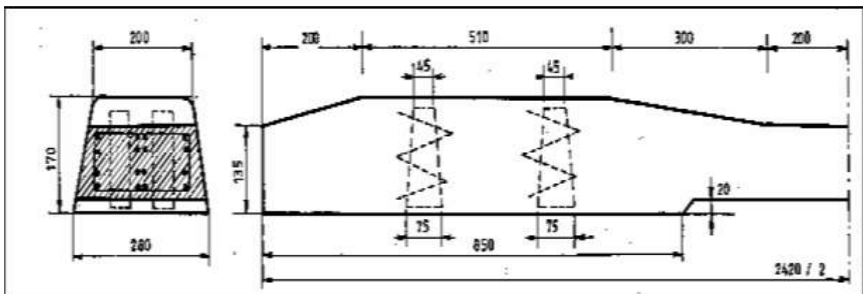
„H” – jelű vasbetonalj (1958-1965)
