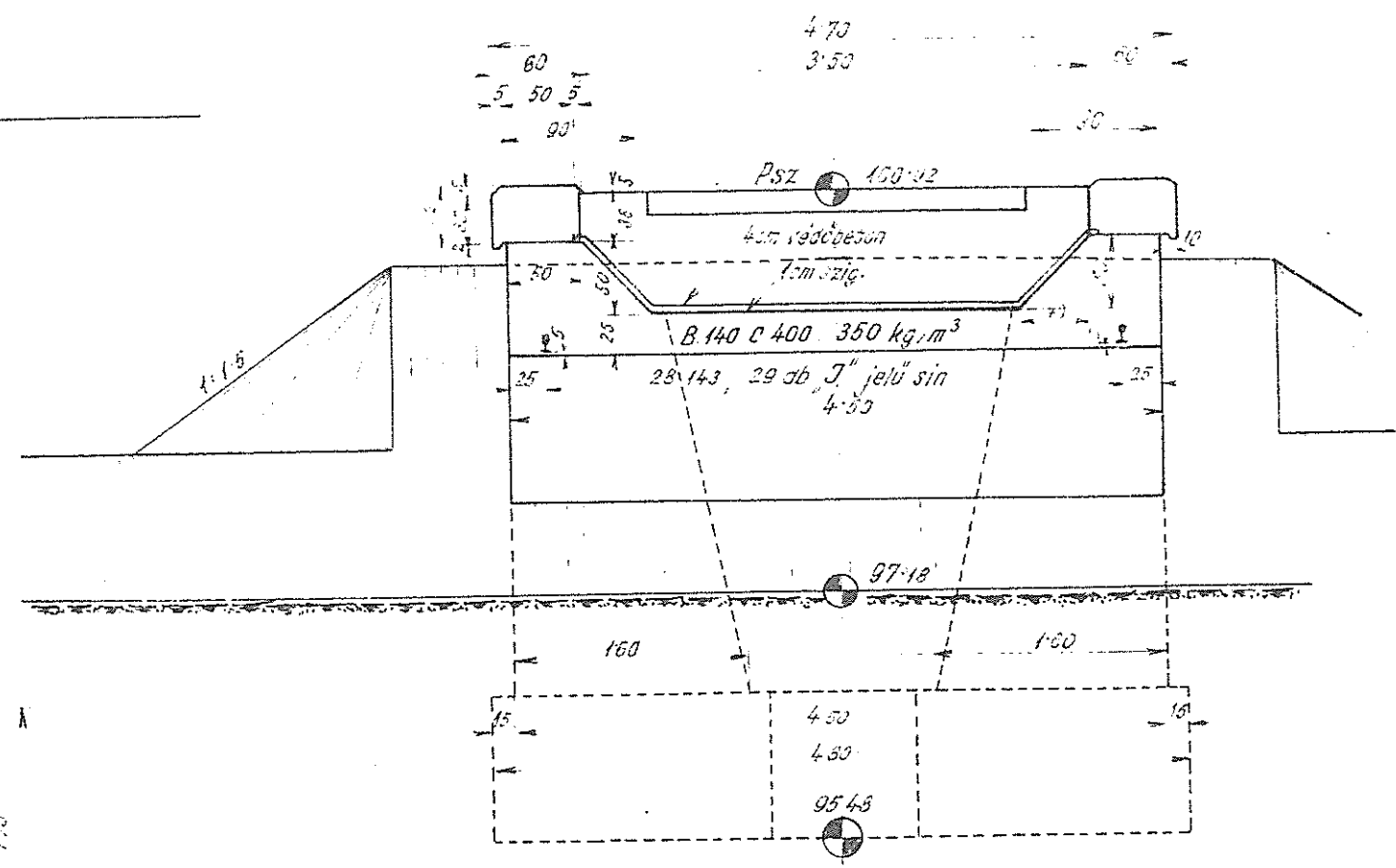
Keresztmetszet
