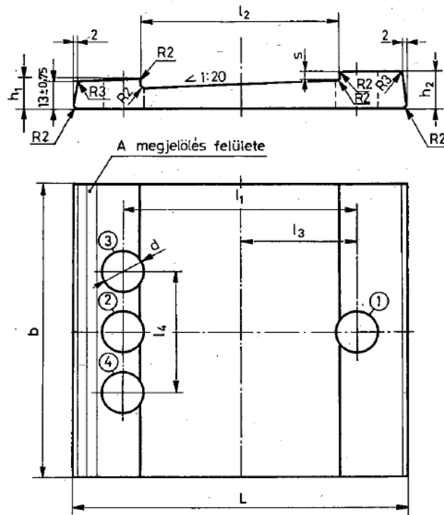
4. ábra Egyszerű nyitott alátétlemez, 1/20 hajlású (típuszám: 34–581, 34–582, 34–583)
