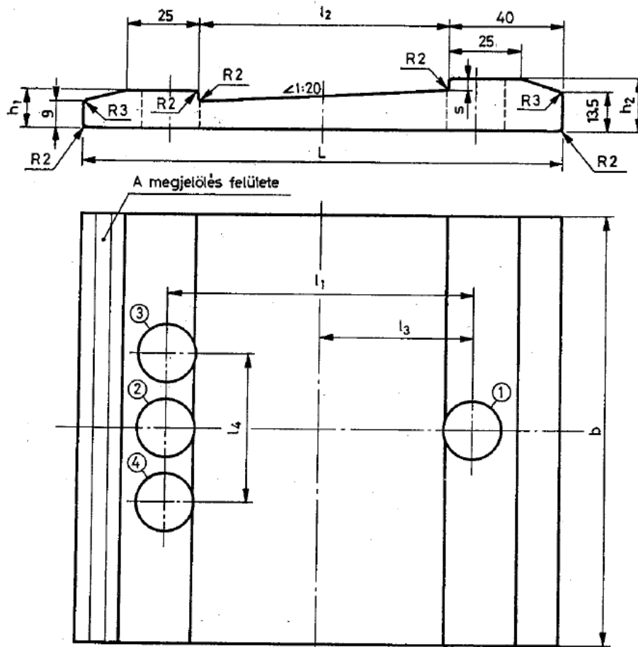
5. ábra Egyszerű nyitott alátételemez, 1/20 hajlású (típuszám: 23-591, 23-592, 23-593)
