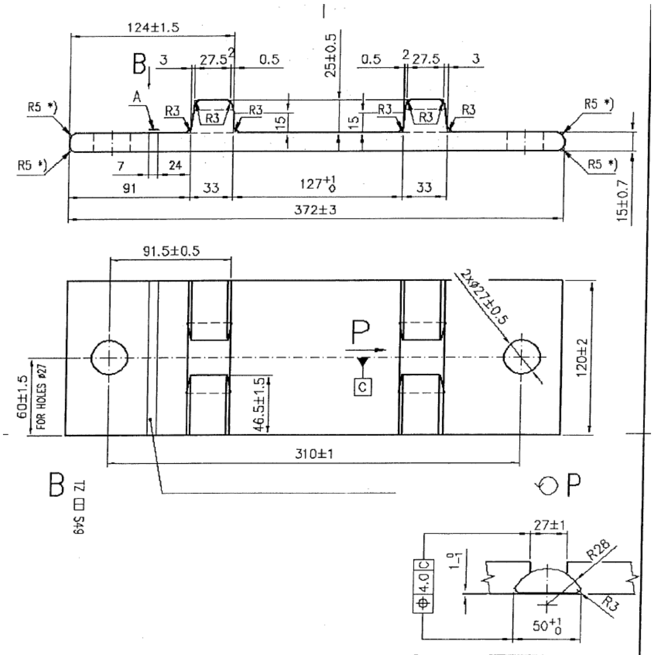
1. sz. rajz S49/48 r. 2 ly. vízszintes GEO alátétlemez
