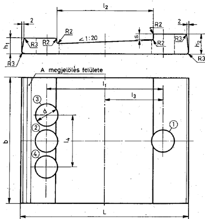
3. ábra Egyszerű nyitott alátétlemez, 1/20 hajlású (típuszám: 54-521, 54-522, 54-523 48-551, 48-553, 48-555)
