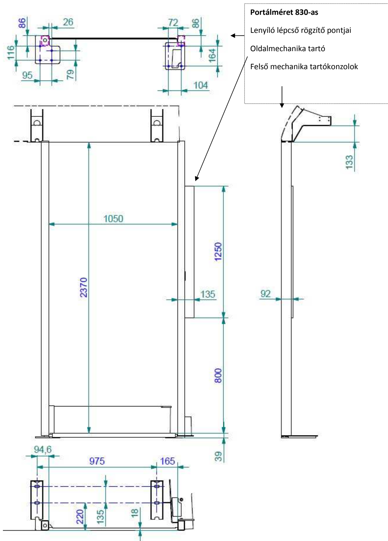
1. ábra: felfogási pontok a kocsiszekrényen 830 mm-es szabad nyílás esetén
