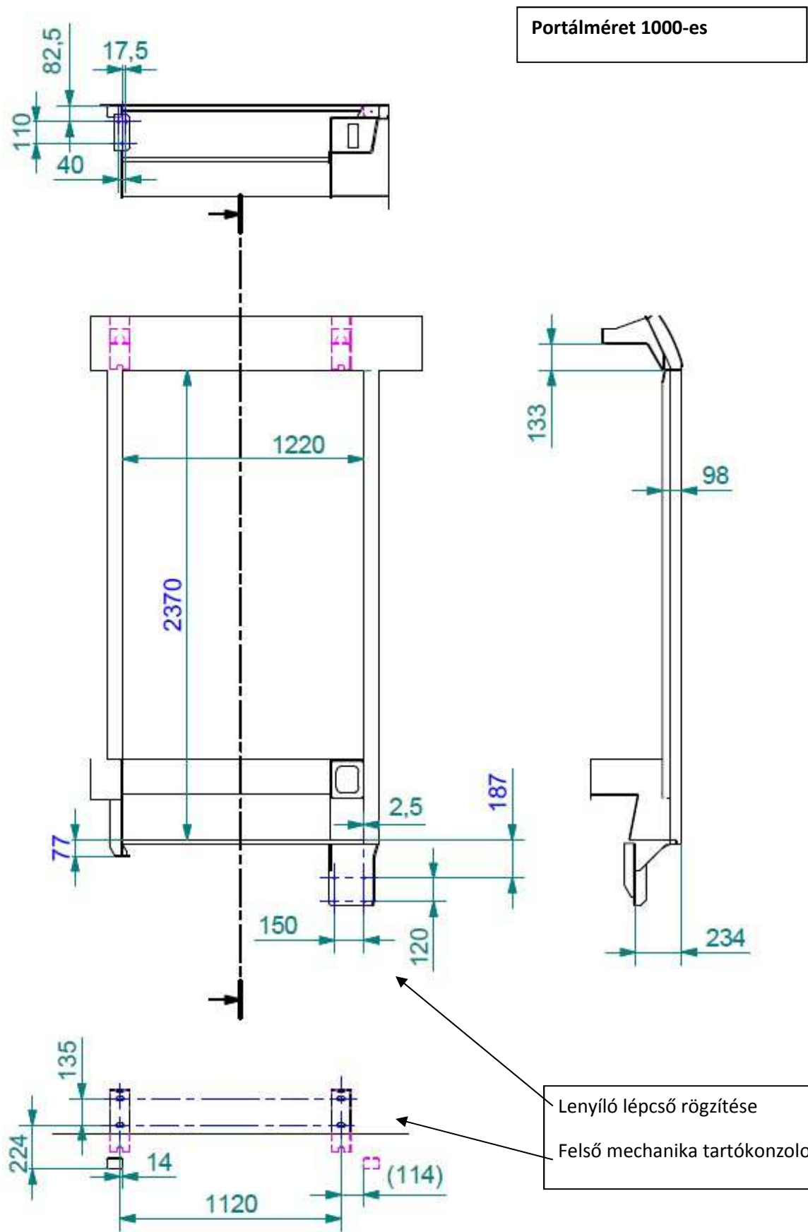
2. ábra: felfogatósi pontok a kocsiszekrényen 1000 mm-es szabad nyílás esetén
