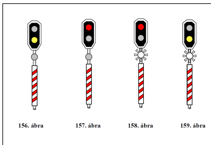
2. sz. ábra: Az F1. utasítás 156-159. ábrája, a mellékvonali ellenőrző jelző
