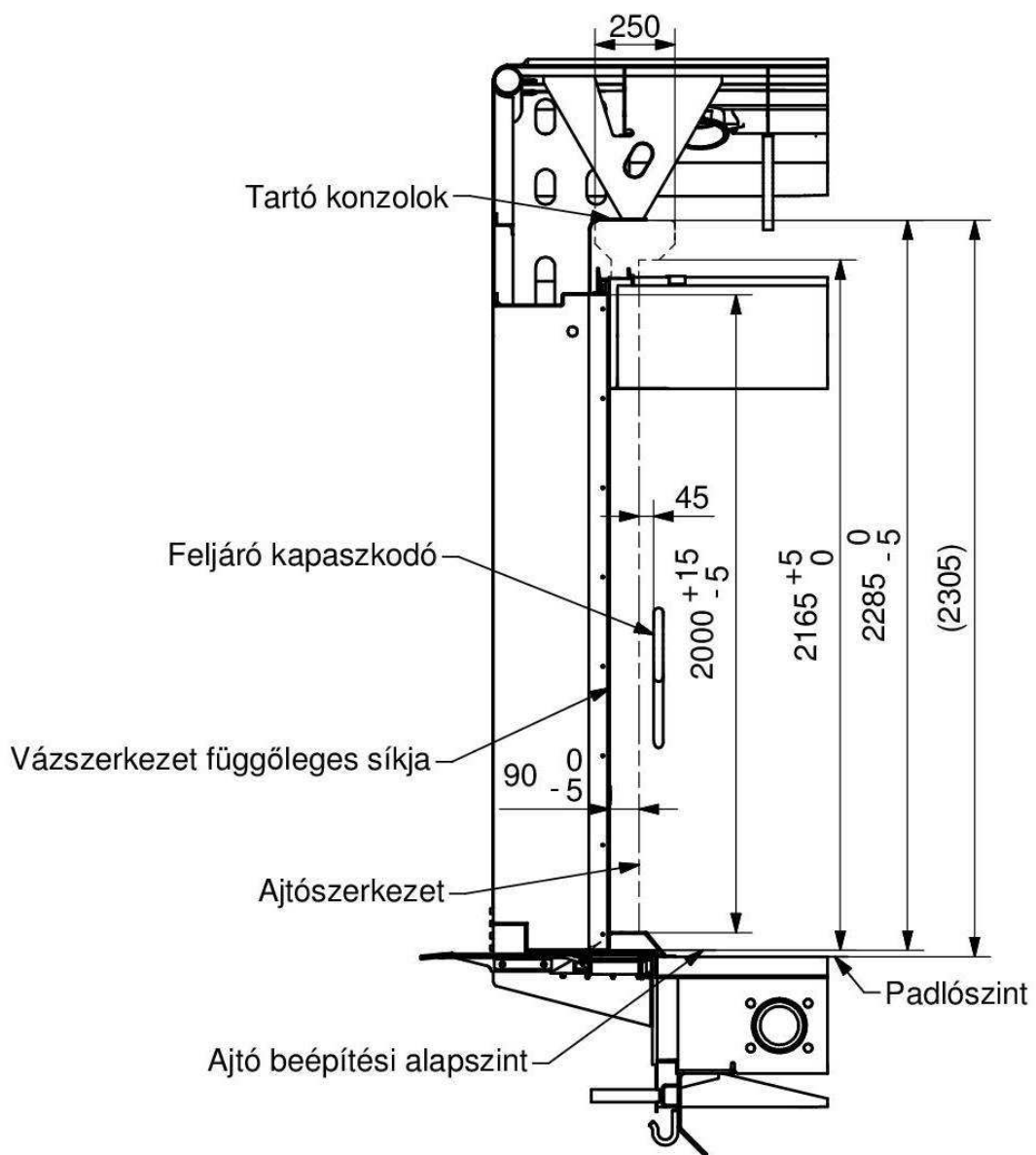
2. ábra Homlok átjáró ajtó beépítési méretek (Kocsi hosszanti metszet)
