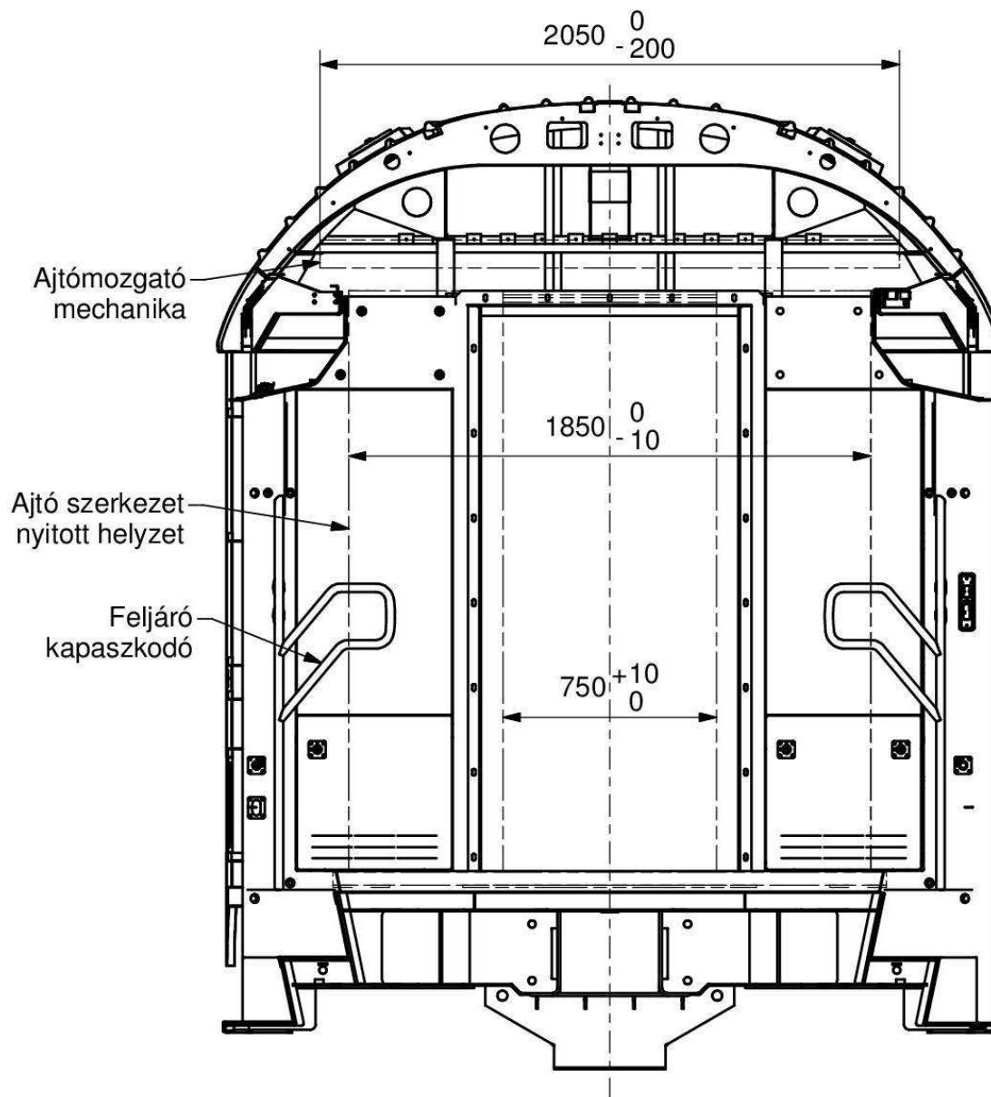
1. ábra Homlok átjáró ajtó beépítési méretek (Ajtó nyitott helyzet)
