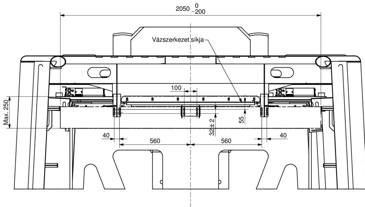
3. ábra Homlok átjáró ajtó beépítési méretek (Rögzítési pontok)
